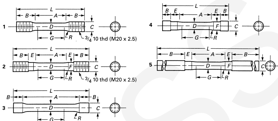
DIMENSIONS
